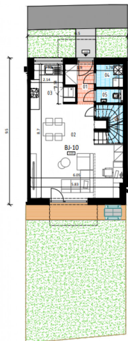
PÔDORYS 1.NP
