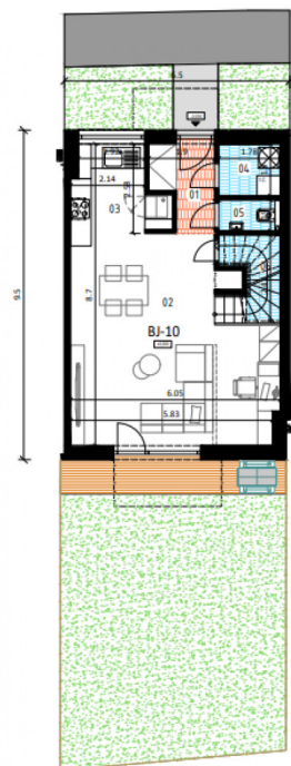
PÔDORYS 1.NP
