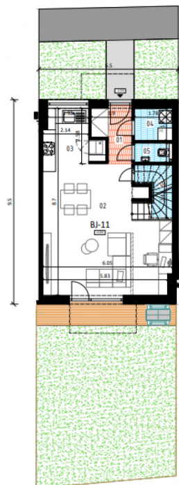
PÓDORYS 1.NP
